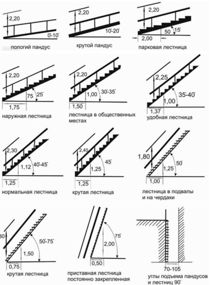
Рис. 1. Нормативные требования по устройству лестниц
